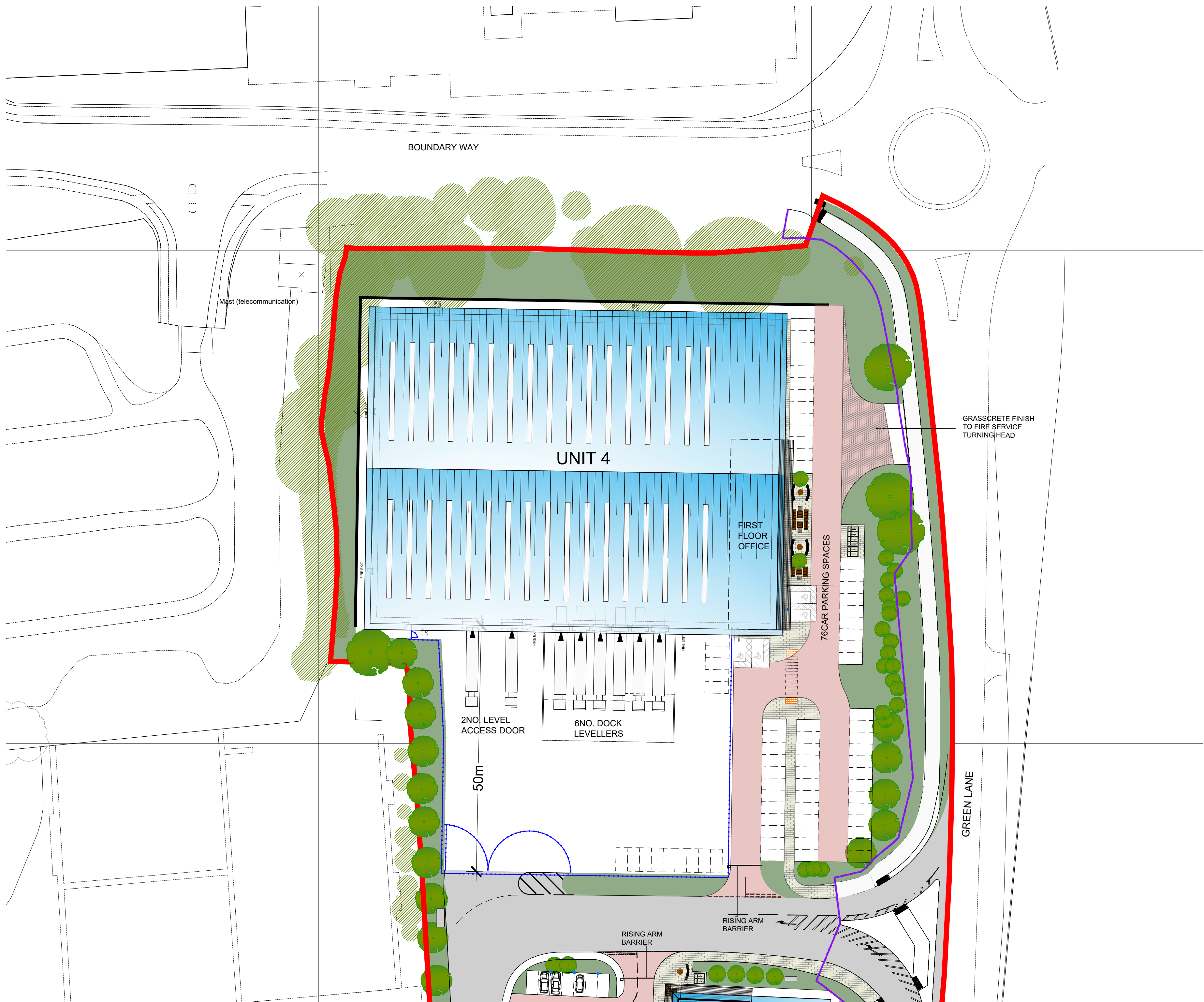
01 214 UNIT 4 SITE LAYOUT 1:500
